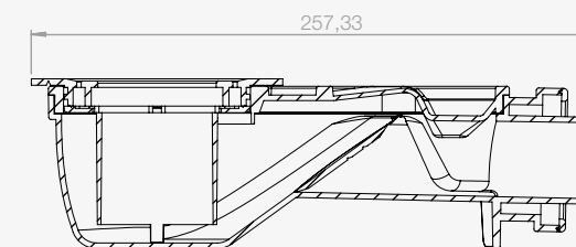
SECCIÓN B-B
