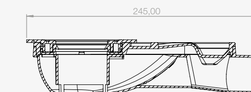
SECCIÓN A-A
